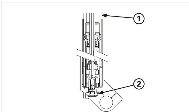
(1) AMMORTIZZATORE DELLA FORCELLA (2) BULLONE CENTRALE DELLA FORCELLA DESTRA
