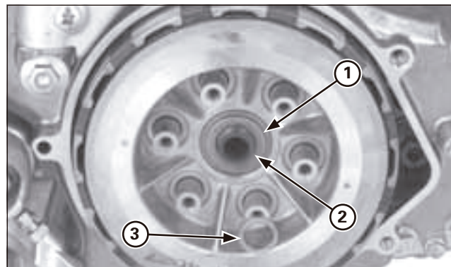
(1) RONDELLA DI SPINTA (2) RONDELLA DI CHIUSURA (SEGNARE "OUTSIDE" DI FRONTE) (3) RONDELLE DI BASE MOLLE
