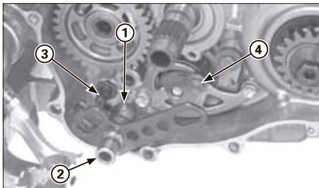
(1) RONDELLA (2) ASSE STRIATO DEL CAMBIO (3) PERNO DELLA MOLLA DI RICHIAMO (4) BOCCOLA DEL SELETTORE
