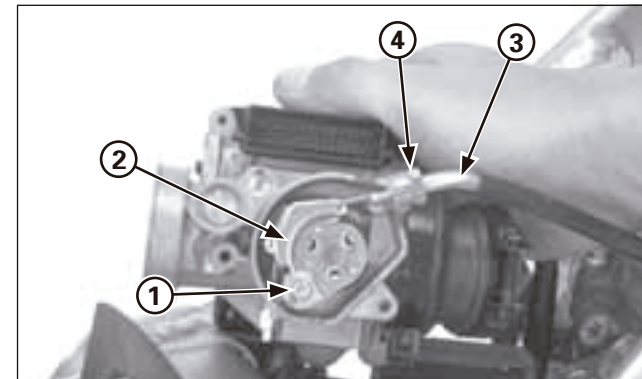
(1) ESTREMIT DEL CAVO DELL'ACCELERATORE (2) TAMBURO DELL'ACCELERATORE (3) CAVO DELL'ACCELERATORE (4) CONTRODADO
