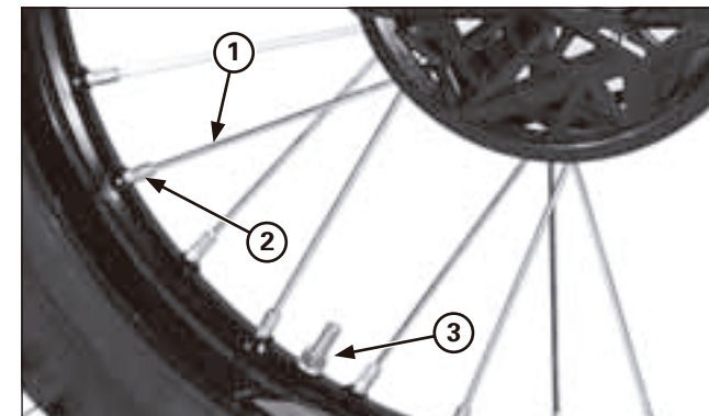
(1) RAGGI (2) DADO DEL RAGGIO (3) CONTRODADO DEL CERCHIO
