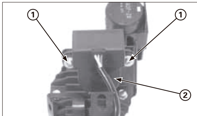
(1) BULLONI (2) SENSORE DELL'ANGOLO D'INCLINAZIONE IN VIRATA
