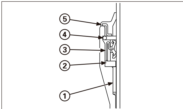
(1) GUIDA DI SCORRIMENTO (2) ANELLO DI SICUREZZA (3) PARAOLIO (4) ANELLO DI FINE CORSA (5) PARAPOLVERE
