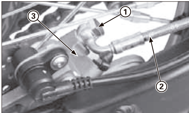
(1) BULLONE DELL'OLIO (2) MANICOTTO DEL FRENO (3) PINZA DEL FRENO
