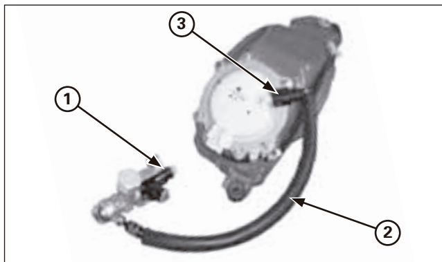
(1) O-RING (NUOVO) (2) TUBO DI ALIMENTAZIONE DEL CARBURANTE (3) CONNETTORE RAPIDO
