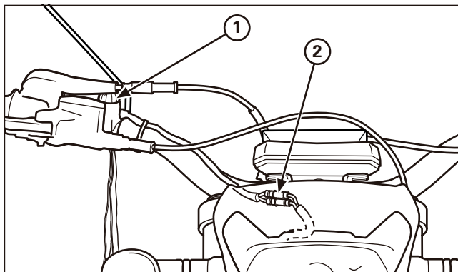
(1) INTERRUTTORE DI ARRESTO MAGNETICO (2) CONNETTORI
