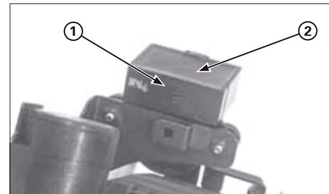
(1) FRECCIA/RIFERIMENTO UP (2) SENSORE DELL'ANGOLO D'INCLINAZIONE IN VIRATA
