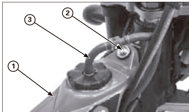
(1) SERBATOIO DEL CARBURANTE (2) BULLONE (3) MANICOTTO DI SFIATO
