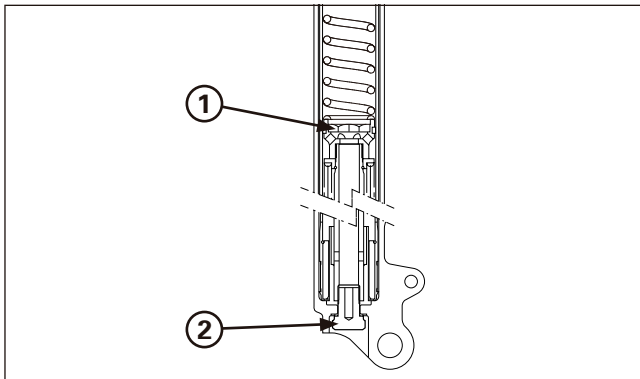
(1) GRUPPO CILINDRO (2) BULLONE CENTRALE
