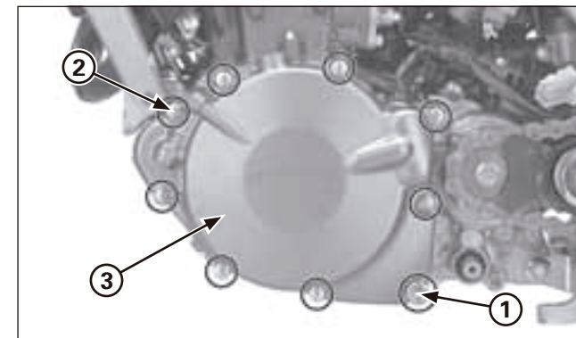
(1) BULLONE DI SCARICO/RONDELLA DI TENUTA (2) BULLONI (3) COPERCHIO DEL CARTER SINISTRO
