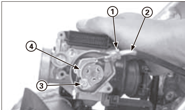
(1) CONTRODADO (2) CAVO DELL'ACCELERATORE (3) ESTREMIT DEL CAVO DELL'ACCELERATORE (4) TAMBURO DELL'ACCELERATORE
