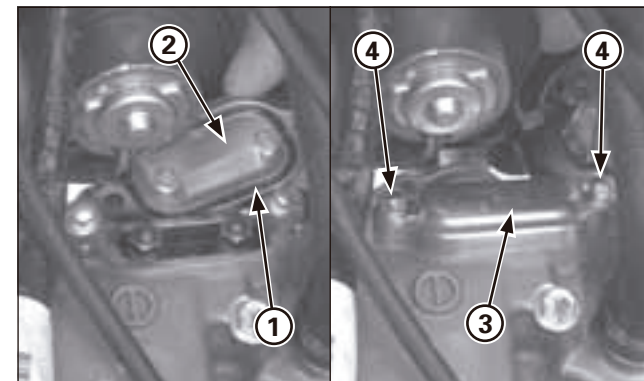
(1) O-RING (2) TAPPO DEL FORO DI REGISTRAZIONE DELLE VALVOLE (3) RIFERIMENTO "UP" (4) BULLONI
