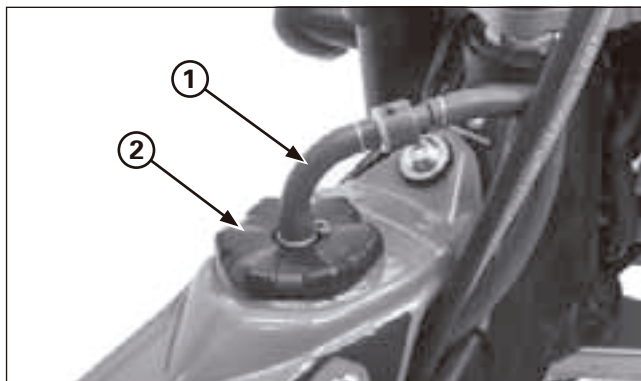
(1) TUBETTO DI SFIATO (2) TAPPO DEL SERBATOIO DI CARBURANTE
