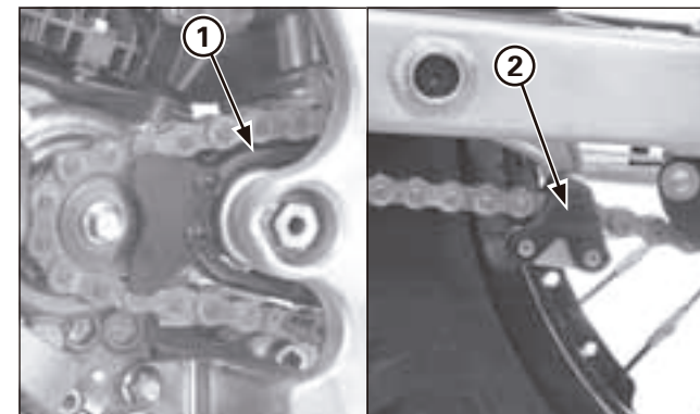
(1) GUIDA DELLA CATENA DI TRASMISSIONE (2) GUIDA DEL TENDICATENA
