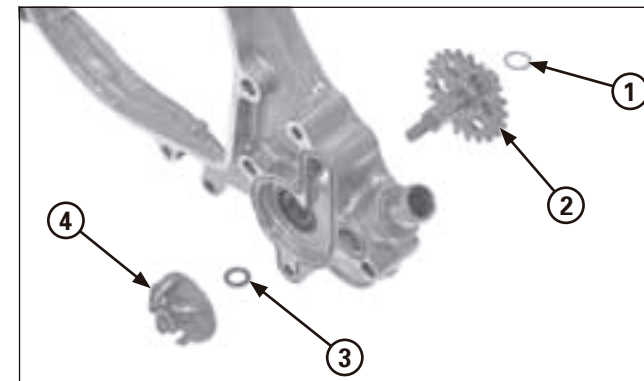
(1) RONDELLE (2) AXE DE LA POMPE EAU (3) RONDELLE NEUVE EN CUIVRE (4) ROTOR
