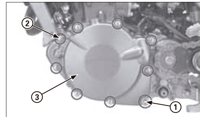
(1) VIS DE VIDANGE/RONDELLE D' TANCH IT (2) VIS (3) CACHE DU CARTER GAUCHE
