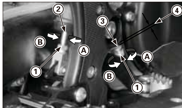
(1) CONTRE- CROU (2) TIGE-POUSOIR (3) VIS DE R GLAGE (4) GARDE
