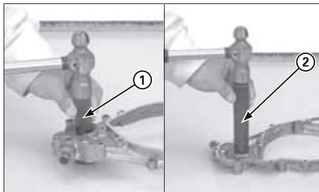
(1) CHASSE-JOINT DE POMPE EAU (2) CHASSE/ACCESSOIRE
