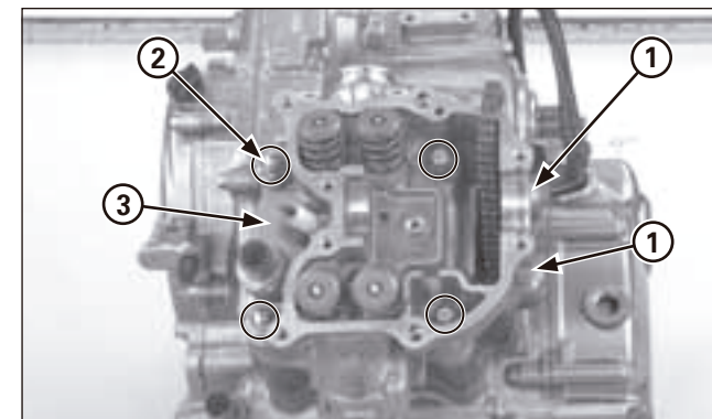
(1) CULASSE (2) RONDELLES/ CROUS (3) VIS
