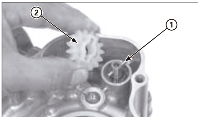
(1) ARBRE MENANT (2) ENGRENAGE MEN DE LA POMPE HUILE
