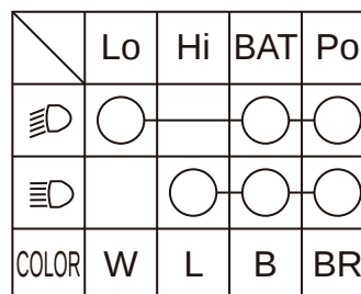
INTERRUPTEUR DES FEUX
