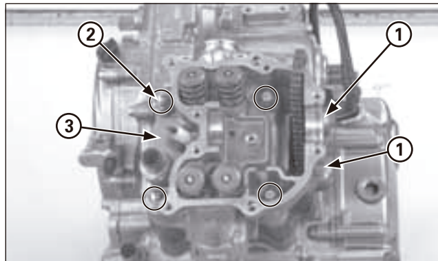
(1) VIS (2) CROUS/RONDELLES (3) CULASSE
