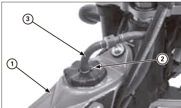
(1) R SERVOIR (2) CLIP (3) DURITE DU RENIFLARD
