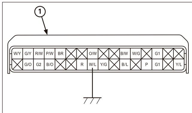
(1) CONNECTEUR 32P INSTALLATION G N RALE
