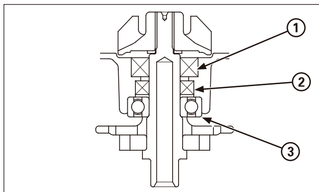
(1) JOINT DE POMPE EAU (2) JOINT D'HUILE (3) ROULEMENT
