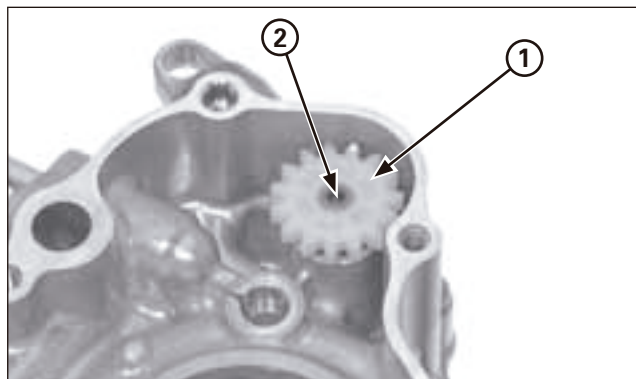
(1) ENGRENAGE MEN (2) AXE DE LA POMPE HUILE
