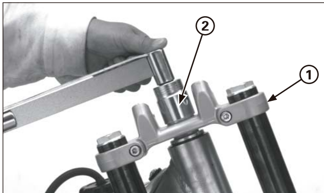
(1) TÊTE SUPÉRIEURE (2) COLONNE DE DIRECTION
