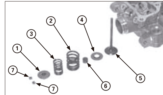
(1) COUVERCLE DU RESSORT DE SOUPAPE (2) RESSORT EXTÉRIEUR (3) RESSORT INTÉRIEUR (4) GUIDE DU RESSORT (5) SOUPAPE (6) BAGUE D'ÉTANCHÉITÉ DE LA SOUPAPE (7) DEMI-FERMETURES
