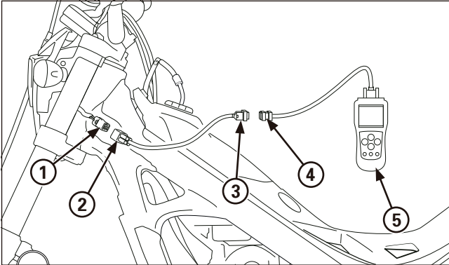
(1) OBD 4P (ROUGE) (2) CONNECTEUR 4P (3) CONNECTEUR 16P (4) OBD CONNECTEUR (5) DST
