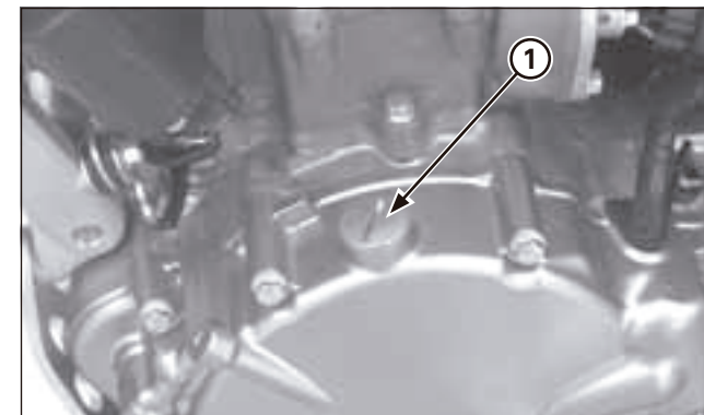
(1) BOUCHON/JOINT TORIQUE DE L'ORIFICE DE REMPLACEMENT
