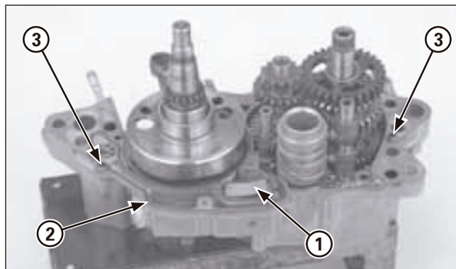
(1) SOUPAPE LAMELLES UNIDIRECTIONNELLE (2) JOINT (3) DOUILLE DE POSITIONNEMENT
