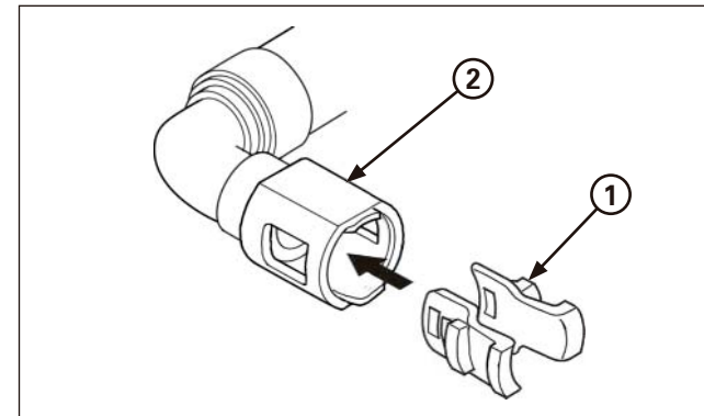
(1) TRIER (2) CONNECTEUR RAPIDE
