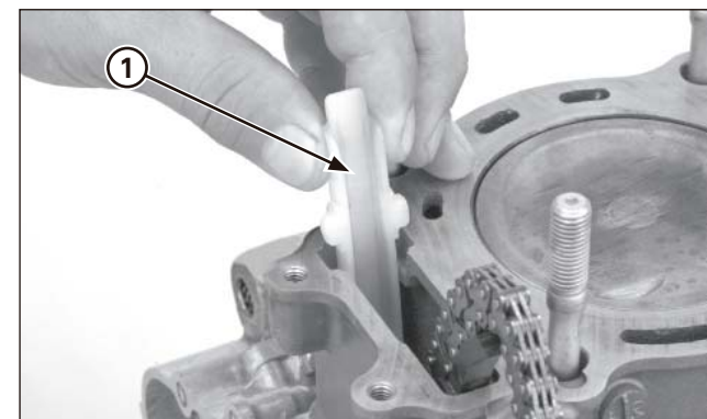
(1) GALET DE GUIDAGE DE LA CHAÎNE DE DISTRIBUTION
