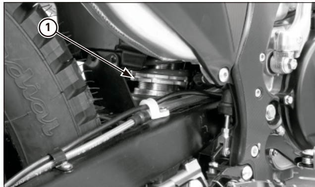
(1) R GULATEUR DE PR CHARGE
