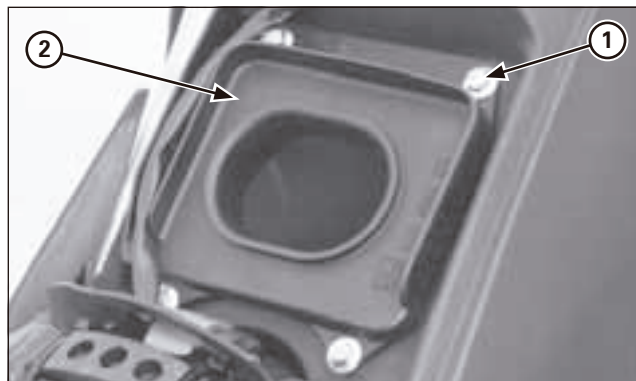
(1) VIS (2) COUVERCLE DU BO TIER DU FILTRE AIR
