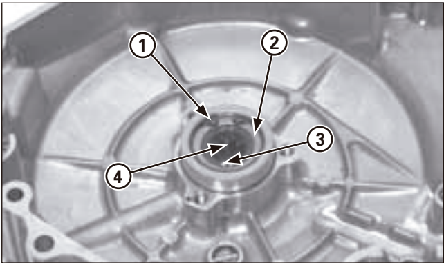
(1) CIRCLIP (2) RONDELLE (3) JOINT D'HUILE (4) ROULEMENT AIGUILLES
