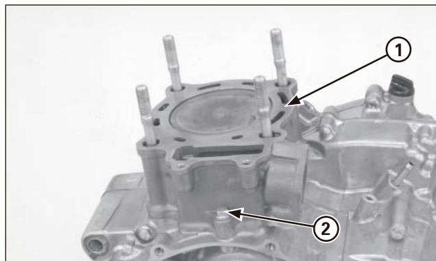
(1) CYLINDRE (2) RONDELLE ET VIS D' TANCH IT NEUVES
