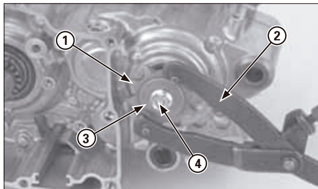
(1) PIGNON DE SORTIE DE BO TE (2) SUPPORT UNIVERSEL (3) ANNEAU RESSORT (4) VIS
