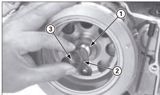
(1) RONDELLE (2) CROU DU VOLANT (3) APPLIQUER DE L'HUILE
