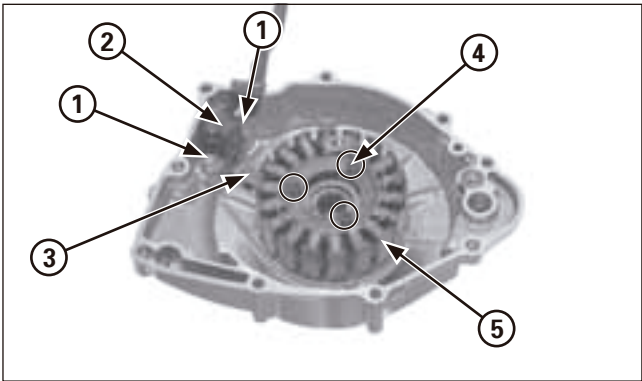
(1) VIS (2) G N RATEUR D'IMPULSIONS D'ALLUMAGE (3) GUIDE-C BLE (4) VIS SIX PANS (5) STATOR
