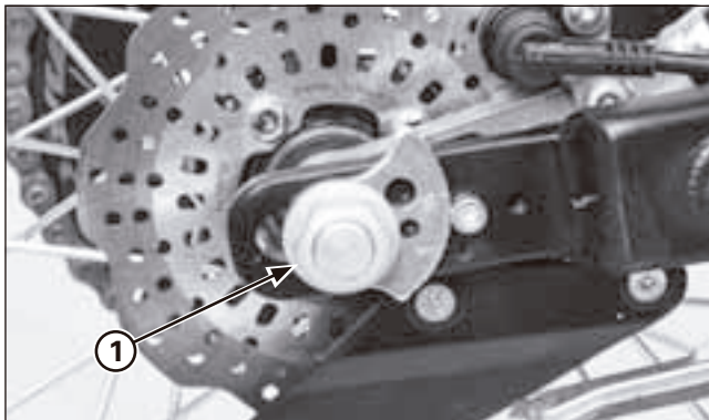
(1) CROU DE L'AXE
