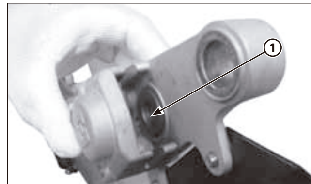
(1) PISTON DE L'ARRIÈRE
