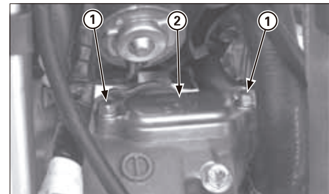
(1) VIS (2) BOUCHON DE L'ORIFICE DE REMPLACEMENT DES CULBUTEURS
