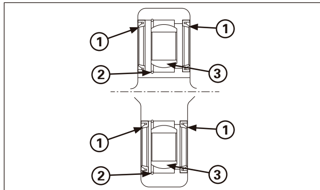
(1) CACHE-POUSSIERE (2) EMBASE DE BUTÉE (2ED/4ED) (3) ROULEMENT SPHÉRIQUE
