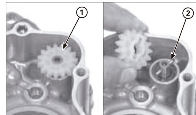
(1) ENGRENAGE MEN (2) ARBRE MENANT
