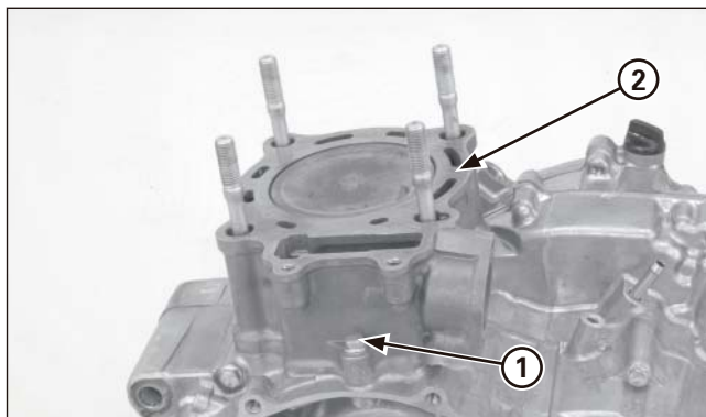
(1) VIS D' TANCH IT /RONDELLE D' TANCH IT (2) CYLINDRE
