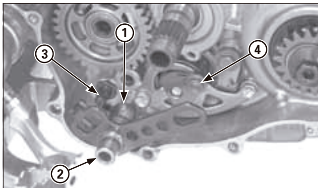
(1) RONDELLE (2) AXE STRI DE LA BO TE DE VITESSES (3) GOUPILLE DU RESSORT DE RAPPEL (4) DOUILLE DE S LECTION
