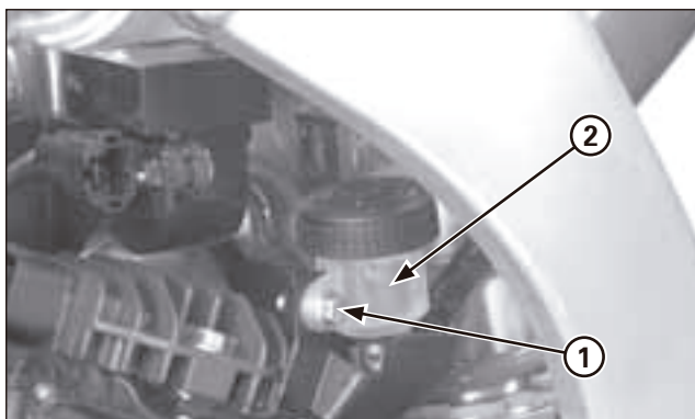
(1) VIS (2) RESERVOIR DE LIQUIDE DE FREIN
