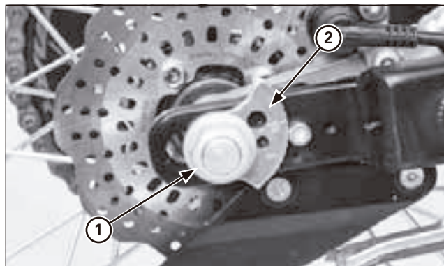
(1) CROU DE L'AXE DE ROUE (2) TENDEUR
