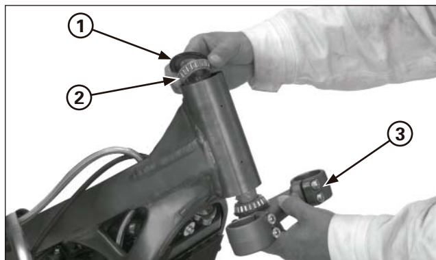
(1) CACHE-POUSSI RE (2) ROULEMENT SUP RIEUR (3) COLONNE DE DIRECTION
