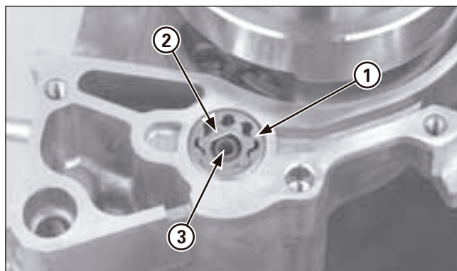
(1) ROTOR EXTERNE (2) ROTOR INTERNE (3) AXE DE LA POMPE HUILE
