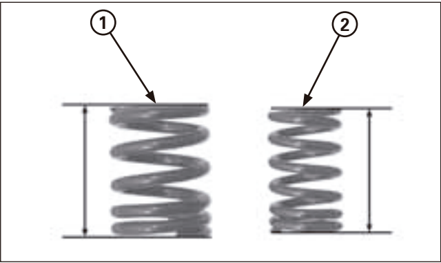
(1) RESSORT DE SOUPEXE EXT RIEUR (2) RESSORT DE SOUPEXE INT RIEUR
