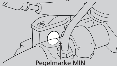
Vorderer Bremsflüssigkeitsbehälter
